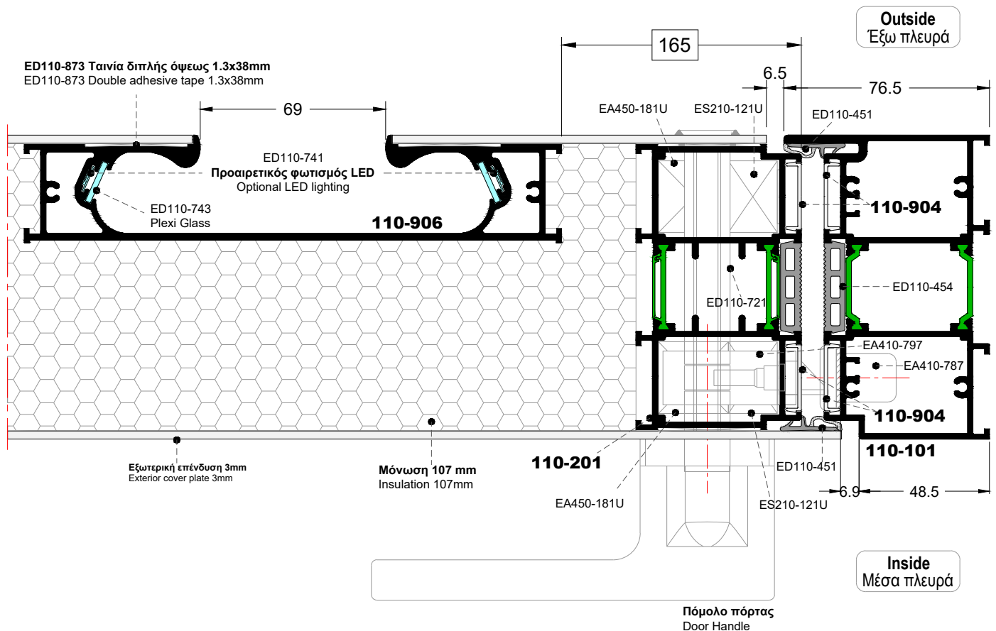
TOP VIEW Κατοψη
