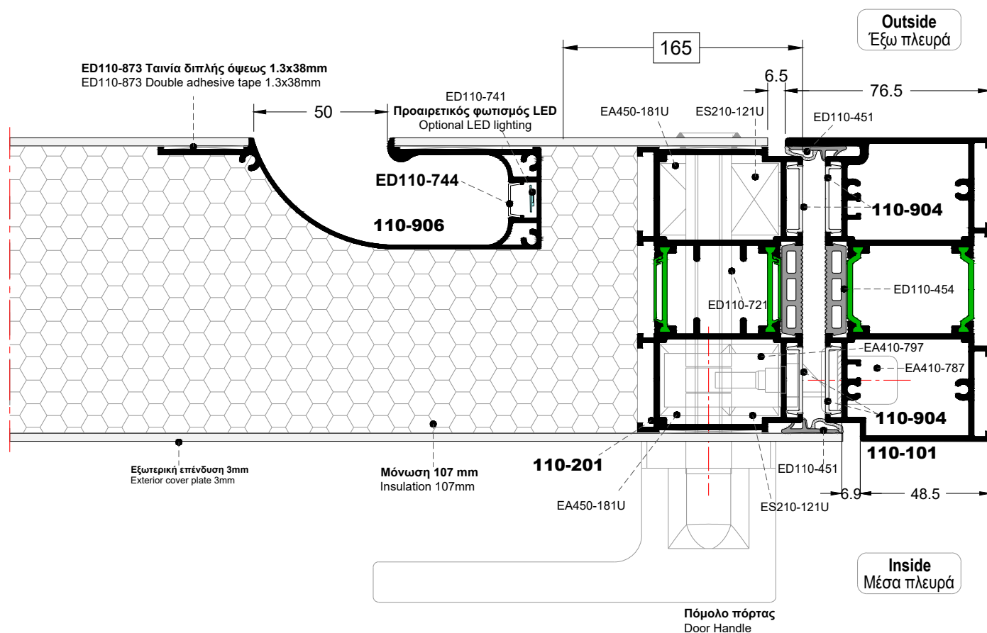
TOP VIEW Κατοψη
