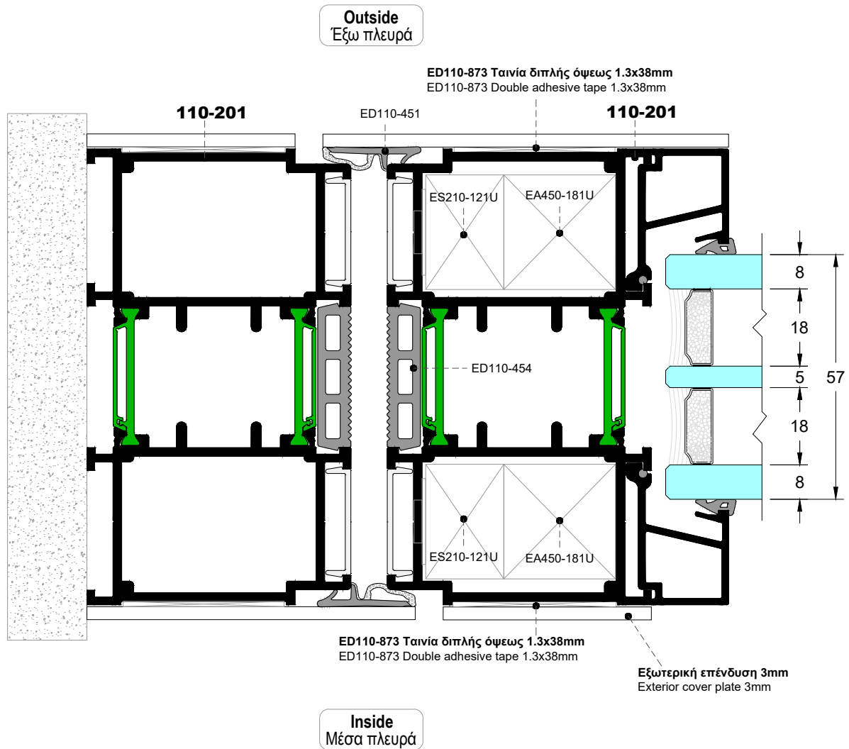
TOP VIEW Κάτοψη
