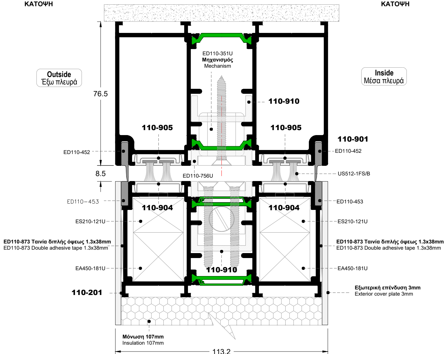
TOP VIEW ΚΑΤΟΨΗ
