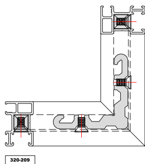
ΛΕΠΤΟΜΕΡΕΙΑ ΚΑΤΕΡΓΑΣΙΑΣ ΓΙΑ 320-209 DETAIL OF MOSQUITO SASH 320-209 DRILLING
