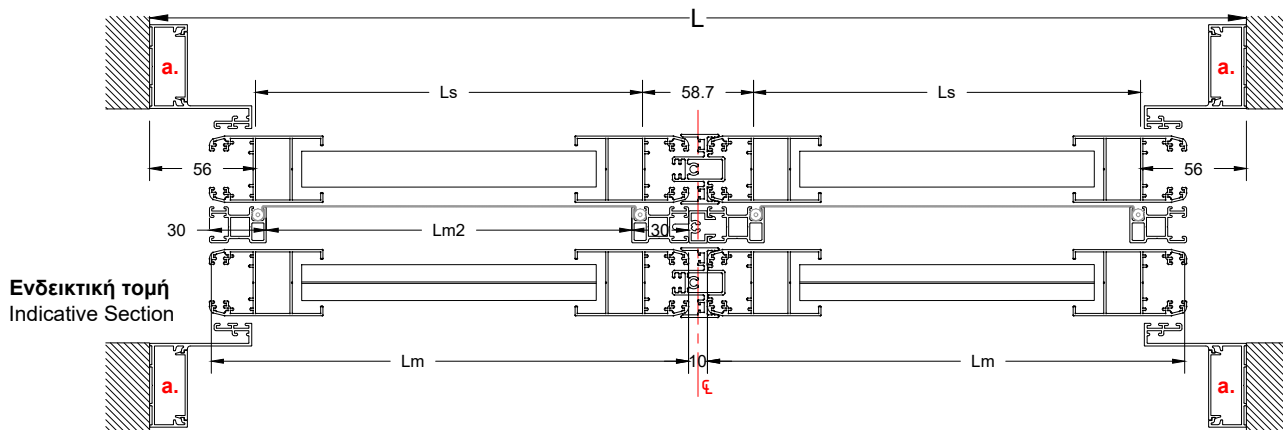
Ενδεικτική τομή Indicative Section
