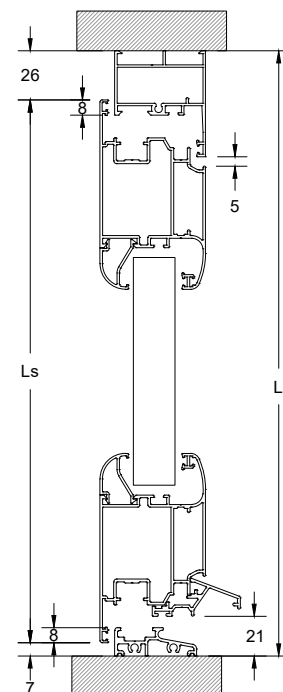
Τζαμιόκι CAMERA ALU 16 Τζαμιόκι CAMERA ALU 16 (περιμετρικός) (περιμετρικός) (Frame 34mm) (Frame 50mm)
