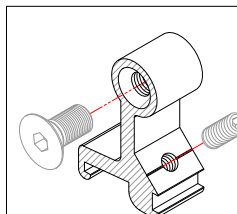
Εσωτερικός σύνδεσμος χωρίσματος Inner connector for transom profile
