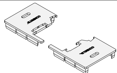
Τάπα φύλλου παντζουριού 540-207 flat Flat end cover for 540-207 sash profile EA540-819M
