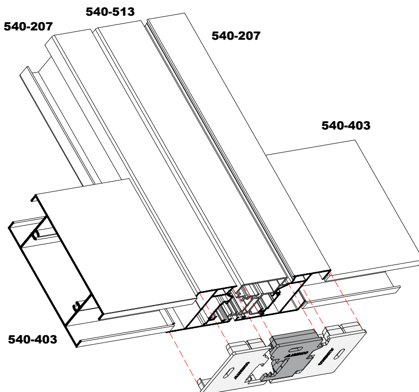
Τάπα φύλλου παντζουριού 540-207 flat Flat end cover for 540-207 sash profile EA540-819M
