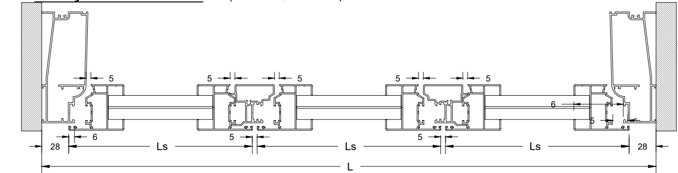
Πατζούρι Τρίφυλλο Triple shutter
