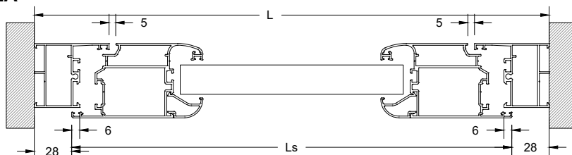
Τζαμιόκι (Camera Europea) Τζαμιόκι (Camera Europea) (Frame 34mm) (Frame 50mm)
