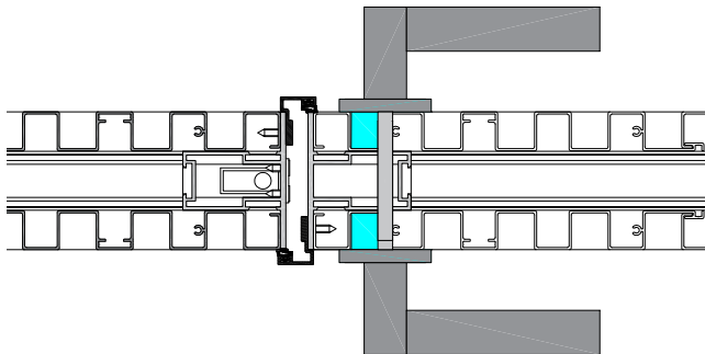
Τομή δίφυλλης ανοιγόμενης αυλόπορτας με χειρολαβή και κρυφό σύρτη Section of double opening gate with handle and latch
