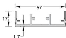
Code/Κωδικός CLS-301 IN STOCK Weight/Βάρος 588 gr/m Length/Μήκος 6 m
