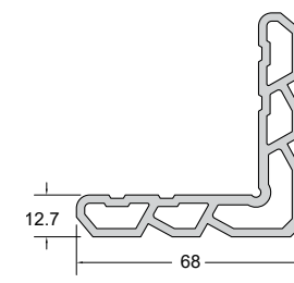
Code/Κωδικός PF031-050 Weight/Βάρος 1995 gr/m Length/Μήκος 6 m Pack/Δέμα 1 Bar/Βέργα
