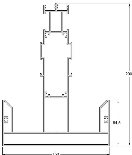
Code/Κωδικός PS20-101 Weight/Βάρος 5889 gr/m Length/Μήκος 4.5 & 6 m
