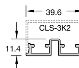
Code/Κωδικός CLS-303 IN STOCK Weight/Βάρος 348 gr/m Length/Μήκος 6 m
