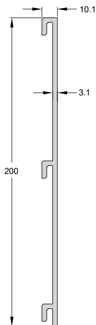
Code/Κωδικός AP20-905 Weight/Βάρος 2050 gr/m Length/Μήκος 6 m
