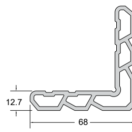
Code/Κωδικός PF031-050 Weight/Βάρος 1995 gr/m Length/Μήκος 6 m Pack/Δέμα 1 Bar/Βέργα
