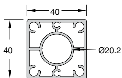
Code/Κωδικός CLS-102 Weight/Βάρος 1245 gr/m Length/Μήκος 6 m
