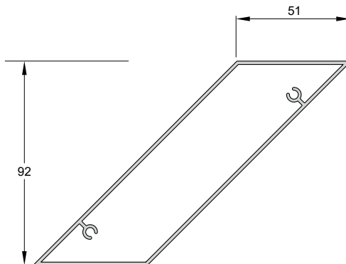
Code/Κωδικός PS10-101 IN STOCK Weight/Βάρος 1554 gr/m Length/Μήκος 6 m Pack/Δέμα 2 Bars/Βέργες
