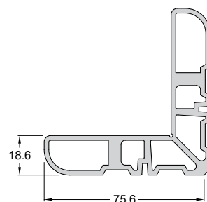
Code/Κωδικός PF31-011 Weight/Βάρος 2622 gr/m Length/Μήκος 6 m Pack/Δέμα 1 Bar/Βέργα
