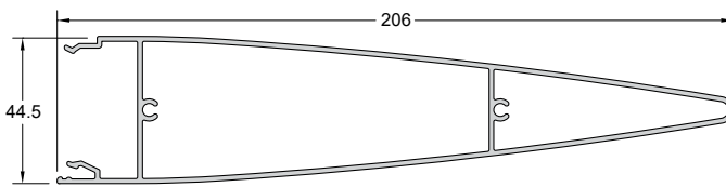
Code/Κωδικός SH3400-212 Weight/Βάρος 2075 gr/m Length/Μήκος 6 m Pack/Δέμα 1 Bar/Βέργα
