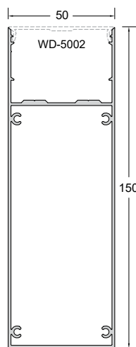
Code/Κωδικός WD-1550 IN STOCK Weight/Βάρος 1611 gr/m Length/Μήκος 6 m Pack/Δέμα 2 Bars/Βέργες
