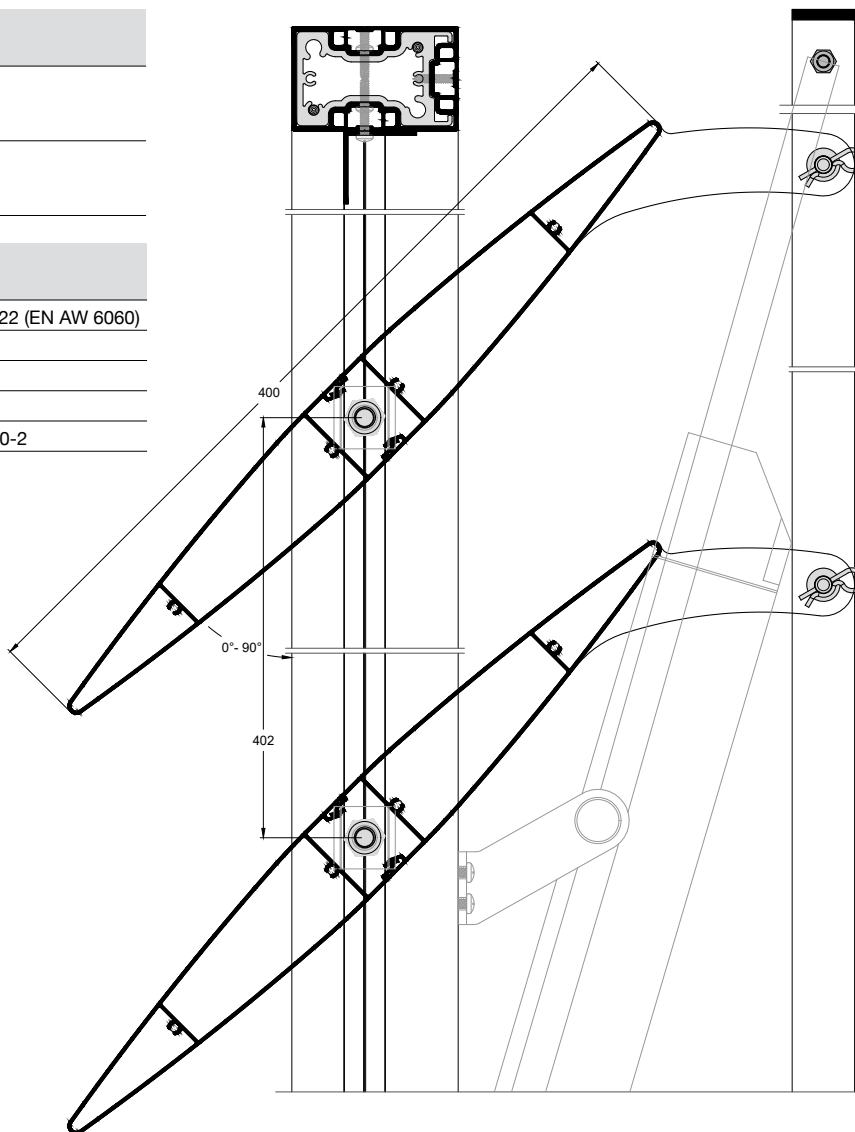
Elliptical design louver with adjustable incline Πτερύγιο ελλειπτικού σχεδιασμού ρυθμιζόμενης κλίσης
