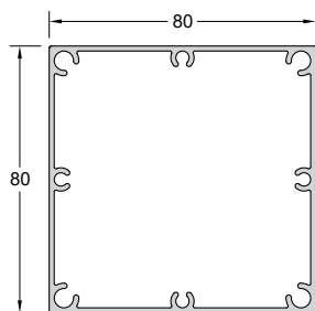
Code/Κωδικός CLS-100 Weight/Βάρος 1606 gr/m Length/Μήκος 6 m
