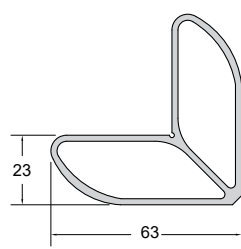
Code/Κωδικός PF31-004 Weight/Βάρος 1417 gr/m Length/Μήκος 6 m Pack/Δέμα 1 Bar/Βέργα
