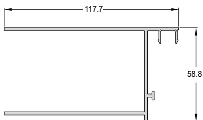
Code/Κωδικός PS20-300 Weight/Βάρος 1540 gr/m Length/Μήκος 4.5 m
