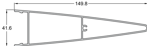
Code/Κωδικός SH3400-206 Weight/Βάρος 1566 gr/m Length/Μήκος 6 m Pack/Δέμα 1 Bar/Βέργα
