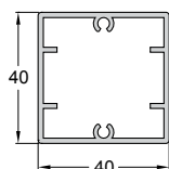
Code/Κωδικός F50-106 Weight/Βάρος 794 gr/m Length/Μήκος 5.8 m
