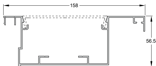
Code/Κωδικός PS20-301 Weight/Βάρος 1534 gr/m Length/Μήκος 4.5 m
