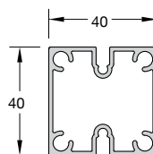
Code/Κωδικός CLS-103 Weight/Βάρος 945 gr/m Length/Μήκος 6 m
