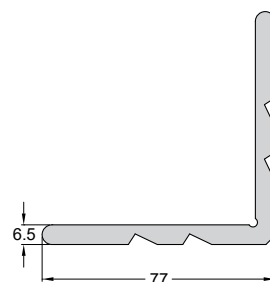
Code/Κωδικός PF31-042 Weight/Βάρος 2364 gr/m Length/Μήκος 6 m Pack/Δέμα 1 Bar/Βέργα
