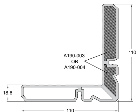
Code/Κωδικός AP110-186 Weight/Βάρος 3378 gr/m Length/Μήκος 6 m Pack/Δέμα 1 Bar/Βέργα
