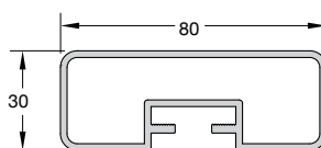
Code/Κωδικός F50-201 Weight/Βάρος 1350 gr/m Length/Μήκος 6 m
