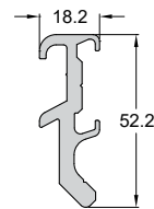
Code/Κωδικός PF31-034 Weight/Βάρος 940 gr/m Length/Μήκος 6 m Pack/Δέμα 1 Bar/Βέργα
