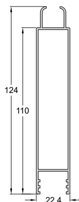
Code/Κωδικός PAT99-045 IN STOCK Weight/Βάρος 1046 gr/m Length/Μήκος 6 m Pack/Δέμα 5 Bars/Βέργες
