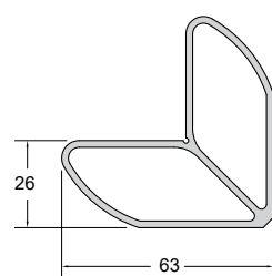
Code/Κωδικός PF31-006 Weight/Βάρος 1335 gr/m Length/Μήκος 6 m Pack/Δέμα 1 Bar/Βέργα
