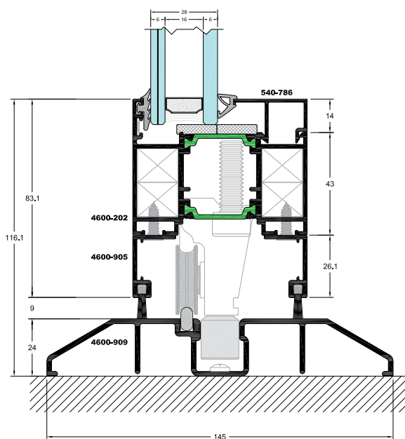
Easy access threshold / Οδηγός εύκολης πρόσβασης
