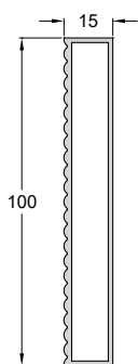
Code/Κωδικός P070-005 IN STOCK Weight/Βάρος 1005 gr/m Length/Μήκος 6 m
