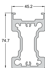
Code/Κωδικός SH3400-951 Weight/Βάρος 2706 gr/m Length/Μήκος 6 m Pack/Δέμα 1 Bar/Βέργα
