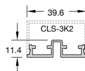
Code/Κωδικός CLS-303 Weight/Βάρος 348 gr/m Length/Μήκος 6 m
