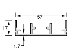
Code/Κωδικός CLS-301 Weight/Βάρος 580 gr/m Length/Μήκος 6 m
