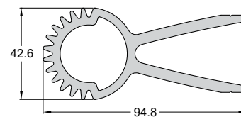
Code/Κωδικός SH3400-905 Weight/Βάρος 2868 gr/m Length/Μήκος 6 m Pack/Δέμα 1 Bar/Βέργα
