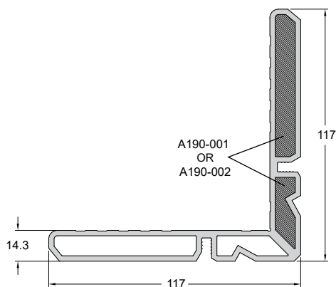
Code/Κωδικός AP110-143 Weight/Βάρος 3336 gr/m Length/Μήκος 6 m Pack/Δέμα 1 Bar/Βέργα
