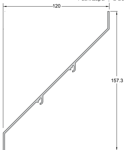
Code/Κωδικός WD-1050 Weight/Βάρος 1260 gr/m Length/Μήκος 6 m Pack/Δέμα 2 Bars/Βέργες
