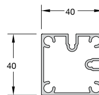
Code/Κωδικός CLS-104 Weight/Βάρος 945 gr/m Length/Μήκος 6 m
