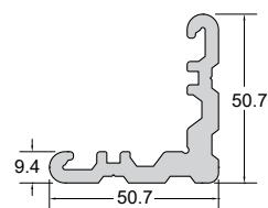
Code/Κωδικός PF31-051 Weight/Βάρος 1607 gr/m Length/Μήκος 6 m Pack/Δέμα 1 Bar/Βέργα
