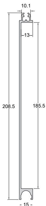
Code/Κωδικός P994-922 IN STOCK Weight/Βάρος 1384 gr/m Length/Μήκος 6 m
