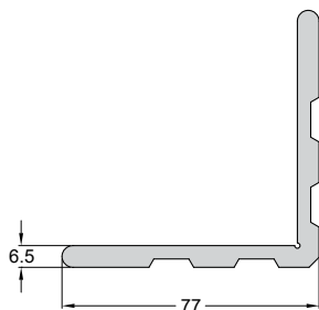
Code/Κωδικός PF31-001 Weight/Βάρος 2225 gr/m Length/Μήκος 6 m Pack/Δέμα 1 Bar/Βέργα
