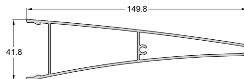
Code/Κωδικός SH3400-207 Weight/Βάρος 1535 gr/m Length/Μήκος 6 m Pack/Δέμα 1 Bar/Βέργα
