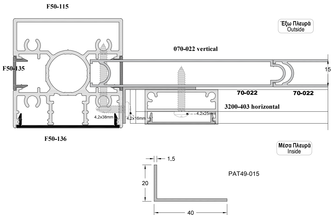
Bottom View ΚΑΤΟΨΗ
