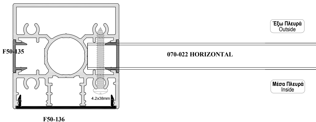
Bottom View ΚΑΤΟΨΗ
