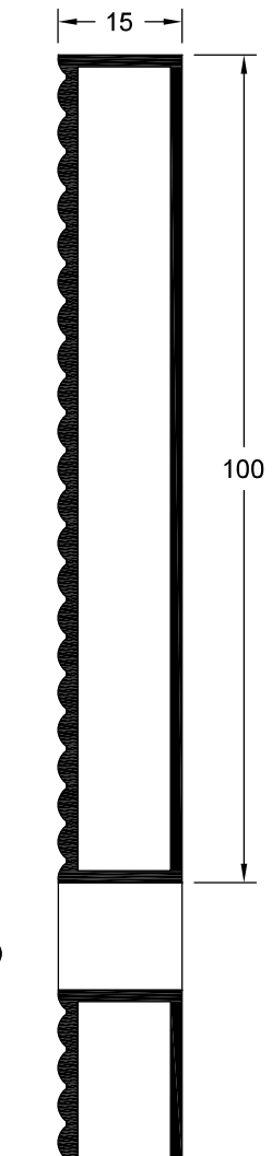
Side View Infill ΠΛΑΓΙΑ ΟΨΗ ΡΑΜΠΟΤΕ
