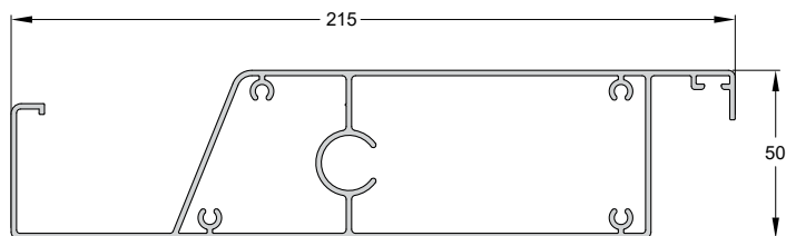
Code/Κωδικός PS20-200 Weight/Βάρος 2740 gr/m Length/Μήκος 4.5, 6 m
