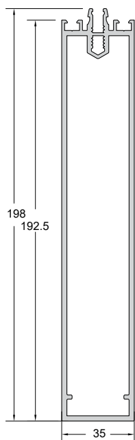
Code/Κωδικός CW35-503 Weight/Βάρος 3296 gr/m Length/Μήκος 6.5 m Pack/Δέμα 1 Bars/Βέργες
