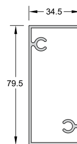
Code/Κωδικός FSN-401 Weight/Βάρος 1142 gr/m Length/Μήκος 6 m
