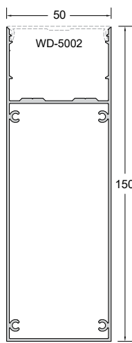
Code/Κωδικός WD-1550 Weight/Βάρος 1611 gr/m Length/Μήκος 6 m Pack/Δέμα 2 Bars/Βέργες
