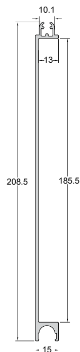
Code/Κωδικός P994-922 Weight/Βάρος 1384 gr/m Length/Μήκος 6 m
