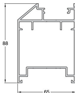
Code/Κωδικός P994-216 Weight/Βάρος 1987 gr/m Length/Μήκος 6 m
