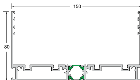
Code/Κωδικός SL55-102 Weight/Βάρος 3210 gr/m Length/Μήκος 6 m
