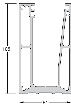
Code/Κωδικός F85-1B65 Weight/Βάρος 3837 gr/m Length/Μήκος 6 m
