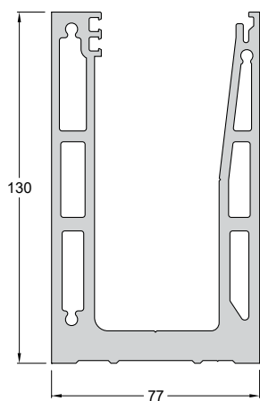
Code/Κωδικός F85-1B63 Weight/Βάρος 7627 gr/m Length/Μήκος 3 m Κατεργασμένο 3.10 m χωρίς κατεργασία
