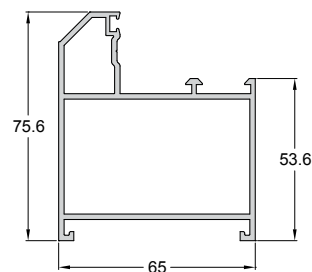
Code/Κωδικός P994-204 Weight/Βάρος 1495 gr/m Length/Μήκος 6 m
