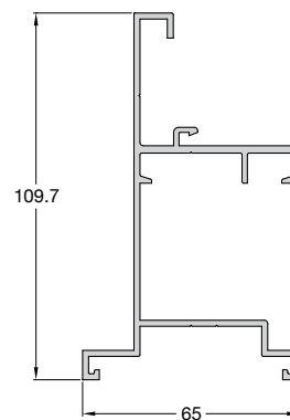
Code/Κωδικός P994-217 Weight/Βάρος 1723 gr/m Length/Μήκος 6 m
