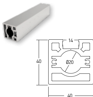
Code/Κωδικός F50-109 Weight/Βάρος 1865 gr/m Length/Μήκος 5.8 m
