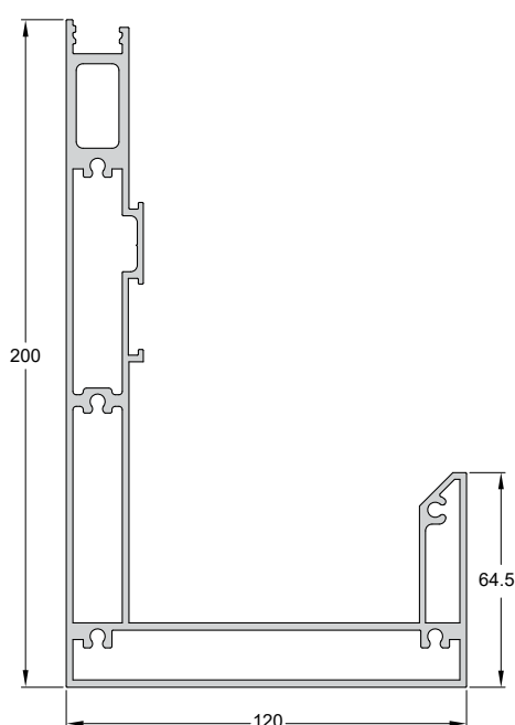
Code/Κωδικός PS20-100 Weight/Βάρος 5044 gr/m Length/Μήκος 4.5, 6 m
