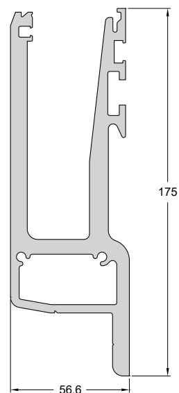
Code/Κωδικός F85-1B69 Weight/Βάρος 7734 gr/m Length/Μήκος 6 m
