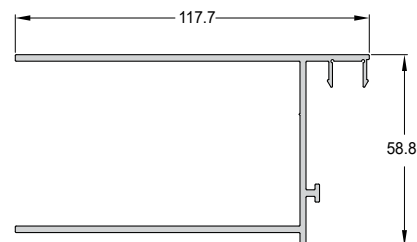
Code/Κωδικός PS20-300 Weight/Βάρος 1540 gr/m Length/Μήκος 4.5 m
