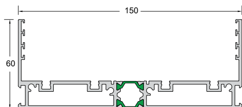
Code/Κωδικός SL55-101 Weight/Βάρος 2957 gr/m Length/Μήκος 6 m
