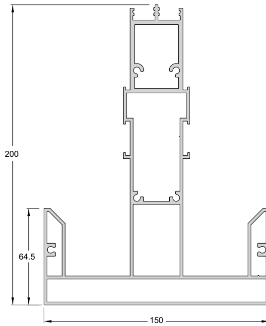
Code/Κωδικός PS20-101 Weight/Βάρος 6275 gr/m Length/Μήκος 4.5 & 6 m
