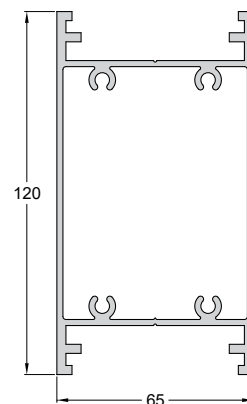
Code/Κωδικός P2050-105 Weight/Βάρος 2503 gr/m Length/Μήκος 6 m
