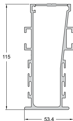
Code/Κωδικός F85-1B74 Weight/Βάρος 2532 gr/m Length/Μήκος 6 m
