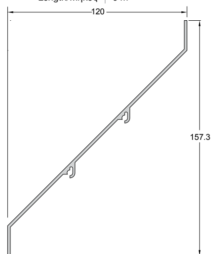
Code/Κωδικός P2050-610 Weight/Βάρος 1163 gr/m Length/Μήκος 6 m
