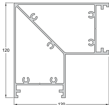
Code/Κωδικός P2050-108 Weight/Βάρος 3575 gr/m Length/Μήκος 6 m
