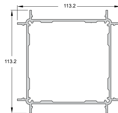
Code/Κωδικός PS20-102 Weight/Βάρος 2975 gr/m Length/Μήκος 3.5 & 6 m
