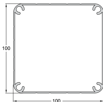
Code/Κωδικός P900-200 Weight/Βάρος 1891 gr/m Length/Μήκος 6 m
