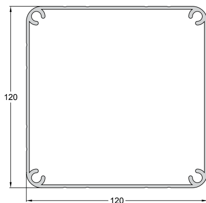
Code/Κωδικός P901-200 Weight/Βάρος 2819 gr/m Length/Μήκος 6 m
