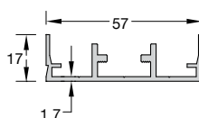
Code/Κωδικός CLS-301 Weight/Βάρος 580 gr/m Length/Μήκος 6 m
