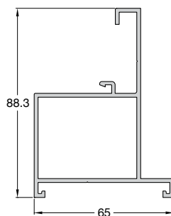
Code/Κωδικός P994-207 Weight/Βάρος 1353 gr/m Length/Μήκος 6 m
