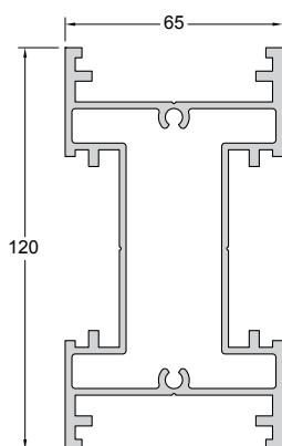
Code/Κωδικός P2050-102 Weight/Βάρος 3075 gr/m Length/Μήκος 6 m
