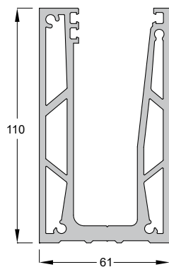
Code/Κωδικός F85-1B75 Weight/Βάρος 5078 gr/m Length/Μήκος 6 m
