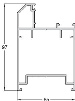
Code/Κωδικός P994-214 Weight/Βάρος 1972 gr/m Length/Μήκος 6 m
