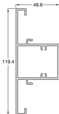
Code/Κωδικός P994-302 Weight/Βάρος 1815 gr/m Length/Μήκος 6 m
