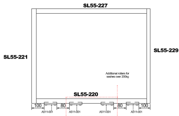
SASH ASSEMBLY FOR VISIBLE SASH TYPOLOGY ΣΥΝΑΡΜΟΛΟΓΗΣΗ ΦΥΛΛΟΥ ΓΙΑ ΤΥΠΟΛΟΓΙΕΣ ΕΜΦΑΝΟΥΣ ΦΥΛΛΟΥ
