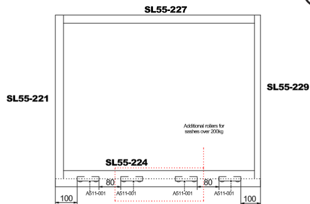
SASH ASSEMBLY FOR HIDDEN TRACK TYPOLOGY ΣΥΝΑΡΜΟΛΟΓΗΣΗ ΦΥΛΛΟΥ ΓΙΑ ΤΥΠΟΛΟΓΙΕΣ ΚΡΥΦΟΥ ΟΔΗΓΟΥ
